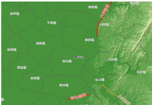
圖 2-2-1、活動斷層圖
